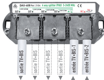
Connexion pour une installation DAU+PAU (2 entrées TV+BIS)
