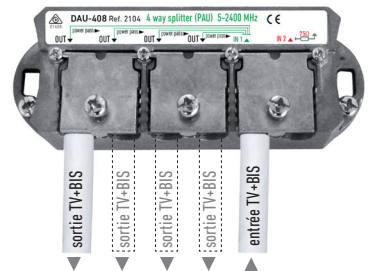
Connexion pour une installation DAU mode répartiteur
