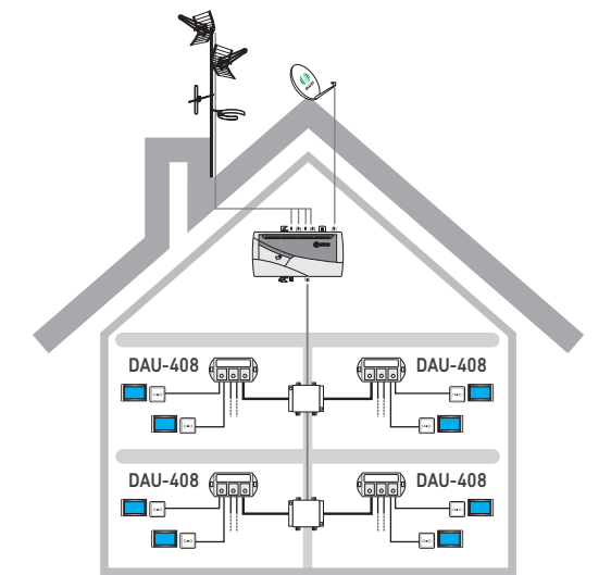
Exemple d'application (mode répartiteur)
