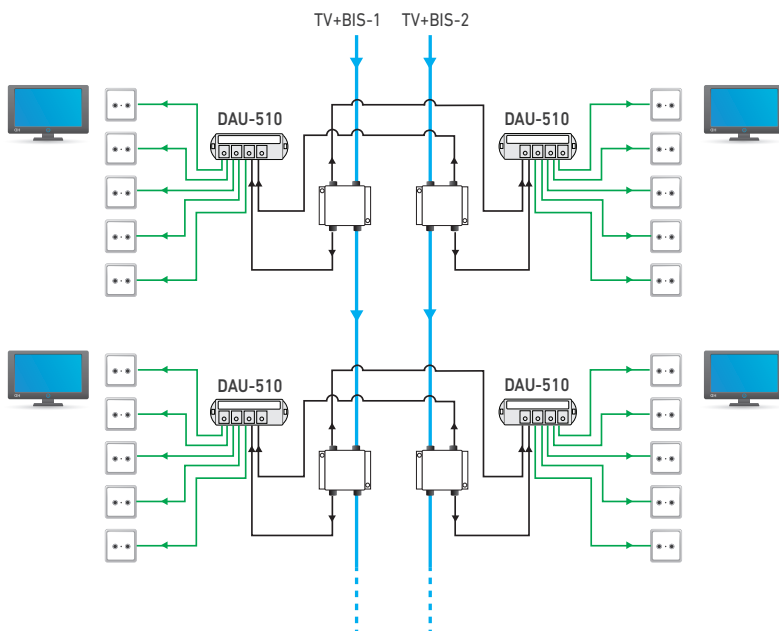
Exemple d'application (mode 2 entrées TV+BIS)
